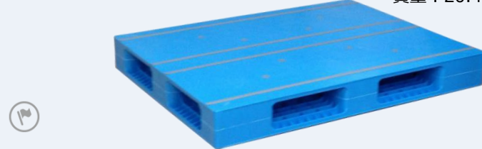
AZFR-1311FE サイズ: 1300×1100×150Hmm 質量: 22.8kg
