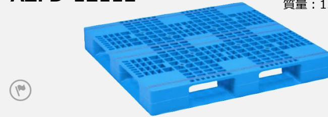
AZFD-1310E サイズ: 1300×1000×150Hmm 質量: 16.1kg
