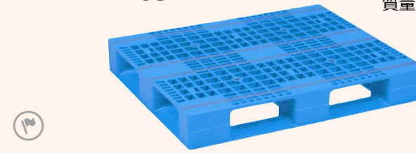
AZFD-1111E サイズ: 1100×1100×150Hmm 質量: 13.3kg
